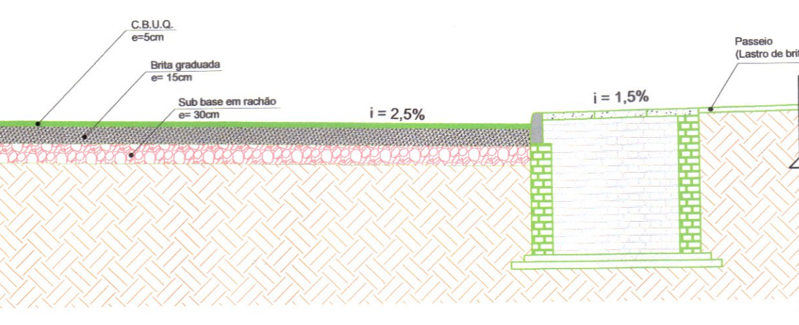
DETALHE ENROCAMENTO EM PEDRAS- INCLINAÇÃO < 45°-LARGURA IGUAL DA BOCA DO BUEIRO SEM ESCALA
